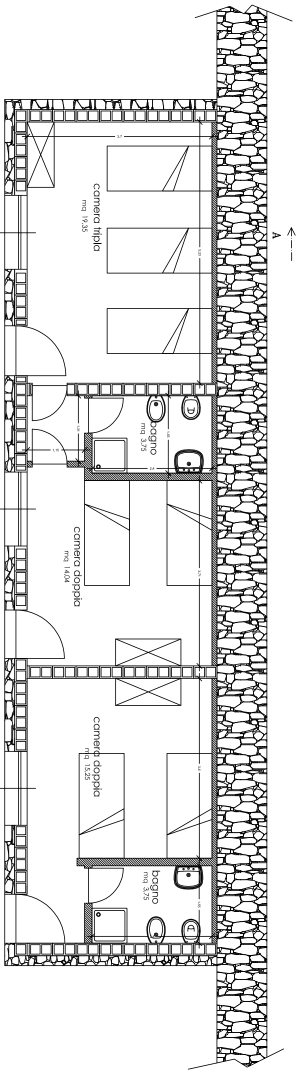
A' Pianta piano terra locali "ex porcellaia"
